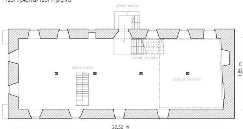
rzut parteru
